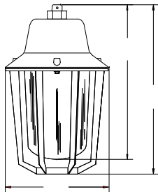
PENDANT MOUNT
